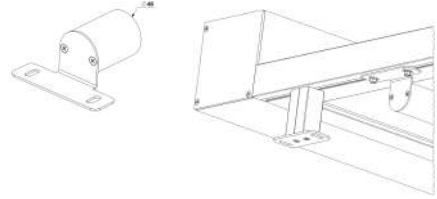
YUVARLAK KILAVUZ BORU
