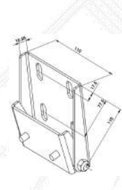
DUVAR BAĞLANTI MAFSALI
