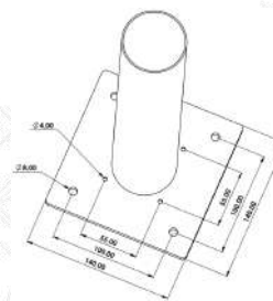
BAĞLANTI AYAĞI
