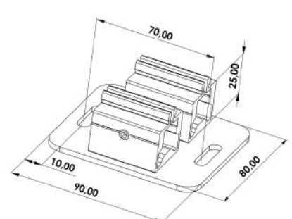
Kiriş Üstü Orta - Büyük Dudaklı Profil
