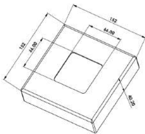
BAĞLANTI KAPAĞI
