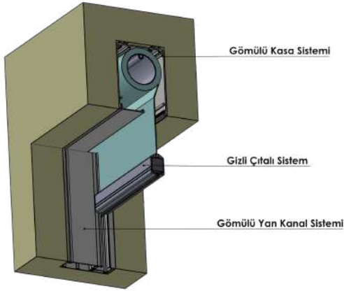
V155r DİKEY GİZLİ ÇITALI VE ALT TAN AÇILABİLİR KAPAKLI ZİP SİSTEMİ
